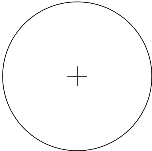
Elementos de la circunferencia
